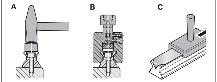
将孔盖或防护带装到滚柱导轨上
