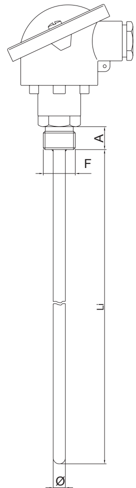
TR6M D con raccordo femmina ed anello saldato
