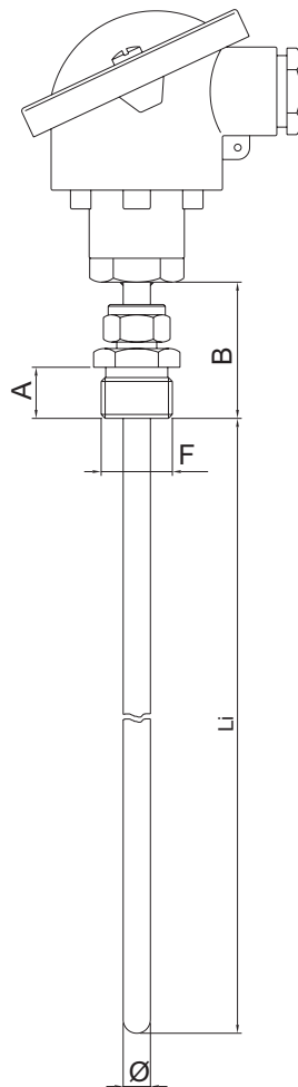
TR6M B con raccordo a compressione scorrevole
