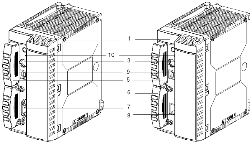
双格式处理器： TSX P57 5634/6634 TSX H57 24M TSX H57 44M
