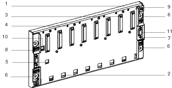
可扩展机架
