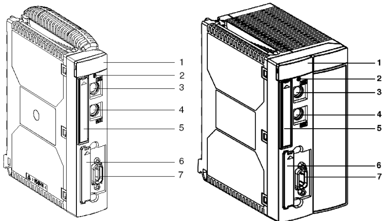
标准格式处理器： TSX P57 0244/104/154
