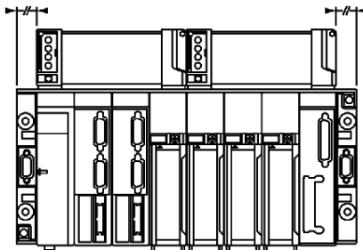
8 位置机架 (TSX RKY 8/8EX)
