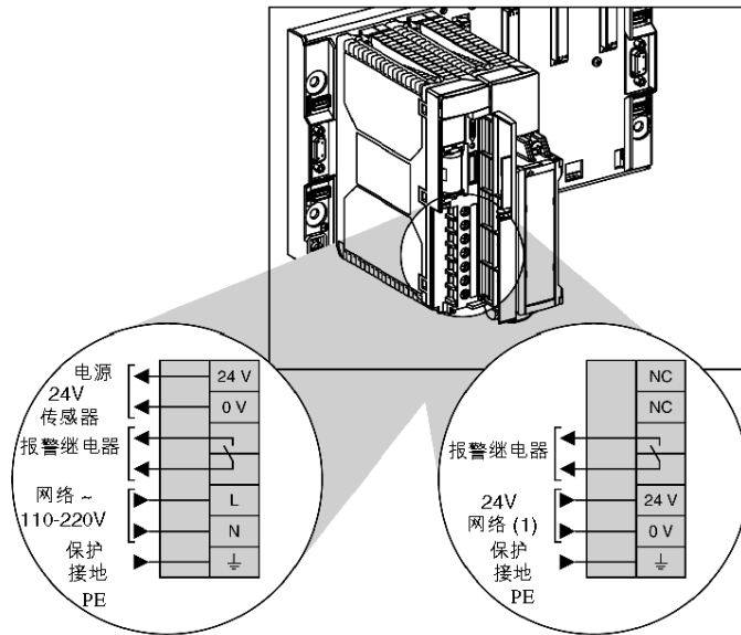
交流电源 TSX PSY 2600/5500/8500
