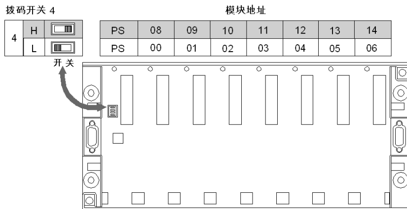
机架 TSX RKY 8EX 上的模块地址示意图
