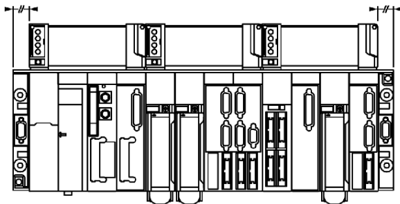
12 位置机架 (TSX RKY 12/12EX)
