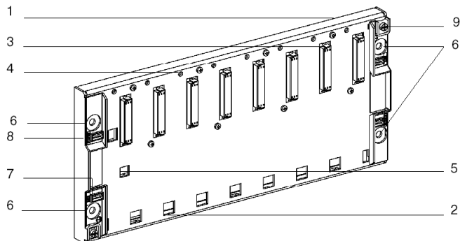
标准机架
