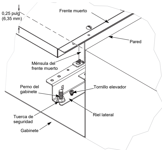
Figura 1: Montaje del interior en gabinetes marca Square D
