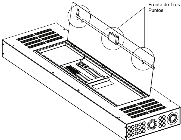
Figure 11: Frente de Tres Puntos
