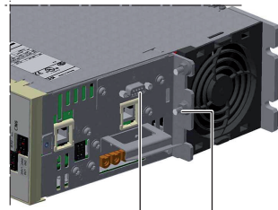
CN12
