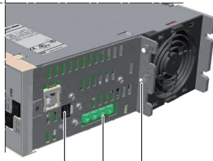
18 18 CN8-1 CN8-2
