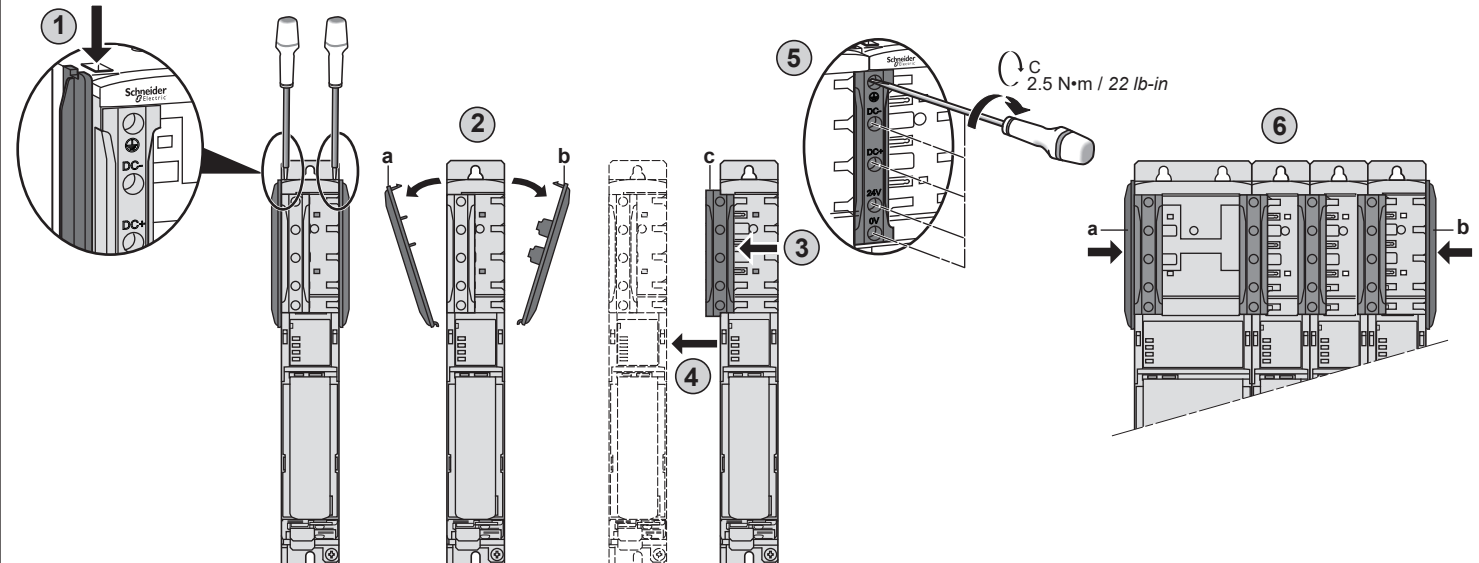
a Shock protector covers left TOP / Capots antichocs gauche HAUT / Stoßsicherungsabdeckungen links OBEN / Cubiertas de protección contra descargas, parte superior izquierda b Shock protector covers right TOP / Capots antichocs droite HAUT / Stoßsicherungsabdeckungen rechts OBEN / Cubiertas de protección contra descargas, parte superior derecha c Bus Bar Module / Module bus barre / Sammelschiene / Módulo de barra de bus / Modulo sbarre / 汇流排模块
