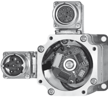
Encoder
