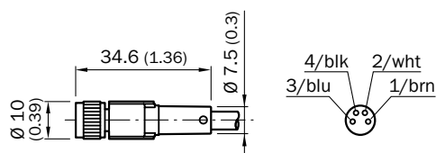
DOL-0804-WxxMC
