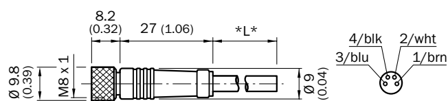
DOL-0804-GxxM
