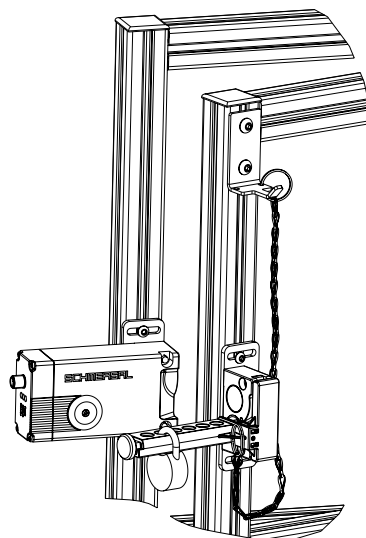
Sblocco con tirante Bowden ACC-AZM400-BOW-M-M
