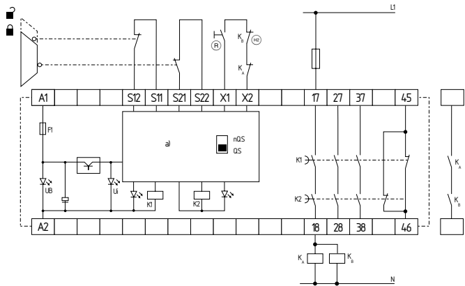
Fig. 4 a) Logic
