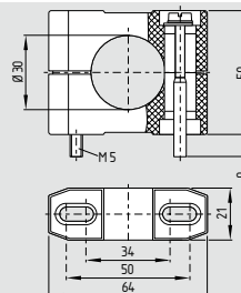
Klemmschelle H 30
