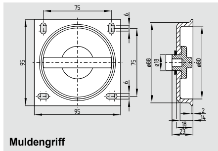
Fluchtentriegelung Metall
