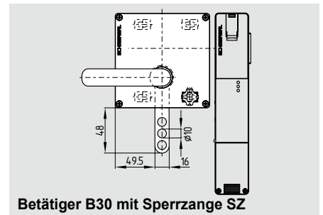
Sperrzange SZ 200-1
