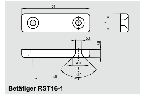
Betätiger RST16-1-R
