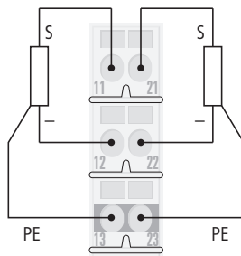
Fig. 175: Wiring diagram BL20-S3x-SBC
