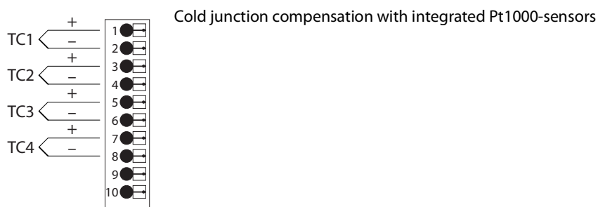
Fig. 158: Wiring diagram
