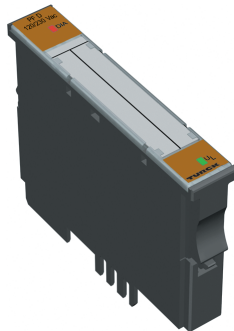
Fig. 32: BL20-PF-120/230VAC-D
