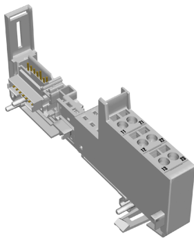
Fig. 117: Base module BL20-S3T-SBB
