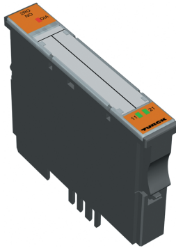
Fig. 235: BL20-2DO-R-NO
