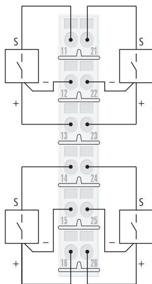
Fig. 68: Wiring diagram BL20-S6x-SBBSBB
