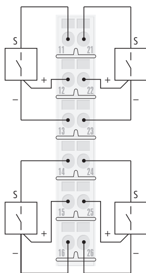
Fig. 74: Wiring diagram BL20-S6x-SBBSBB
