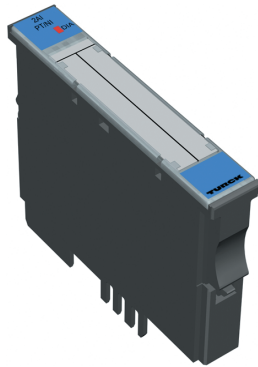
Fig. 130: BL20-2AI-PT/NI-2/3
