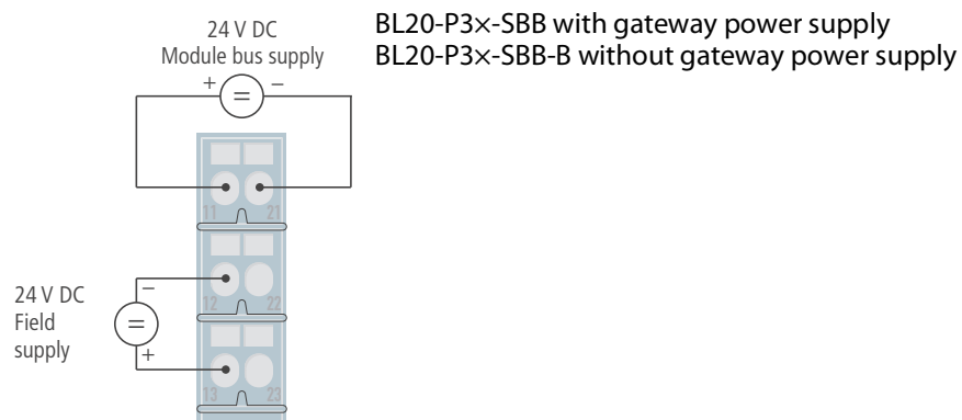
Fig. 43: Wiring diagram
