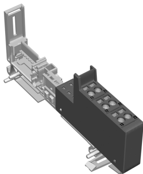
Fig. 28: Base module BL20-P3T-SBB
