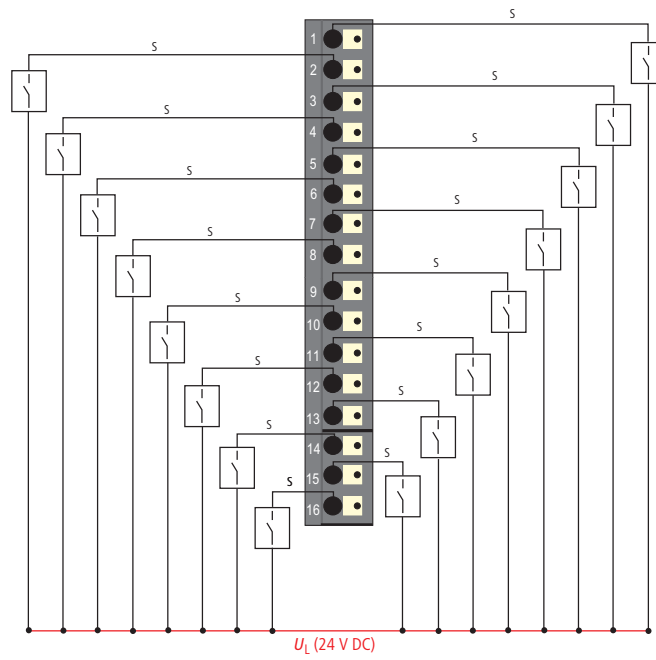
Fig. 91: Wiring diagram
