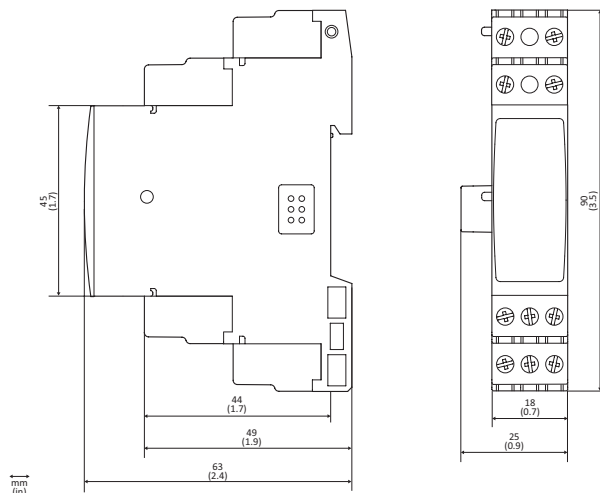
Fig. 2 Dimensioni VMU-OC
