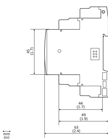
Fig. 1 Dimensioni VMU-MC
