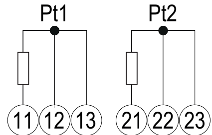
Fig. 8 Temperaturindgange 1 og 2 (3 ledninger)
