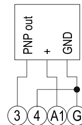
Fig. 16 PNP-impulsindgang (produktkode: 2TCW)
