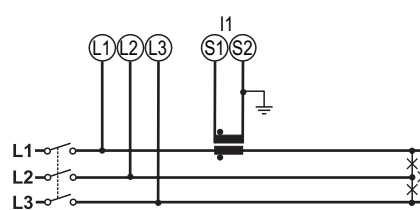
Fig. 11 Trefasesystem uden neutral (3-leder), balanceret belastning, 1 CT.
