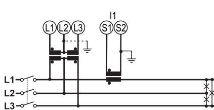
Fig. 12 Trefasesystem uden neutral (3-leder), balanceret belastning, 1 CT og 2 VT/PT.
