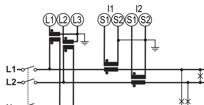
Fig. 14 Tofasesystem (3-leder), 2 CT og 2 VT/PT.
