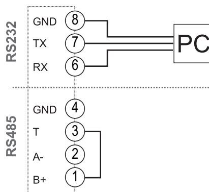
Fig. 21 M C 485232. RS232 seriel port.
