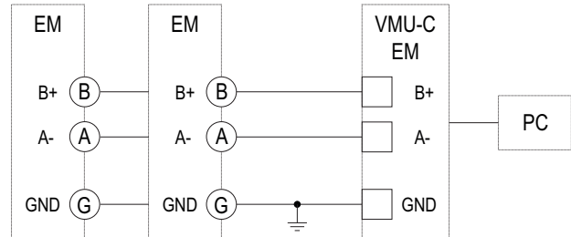
Fig. 2 RS485 COM2 vers compteur d'énergie
