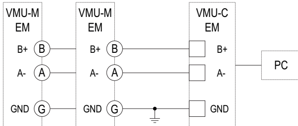
Fig. 1 RS485 COM1 vers modules VMU-M EM
