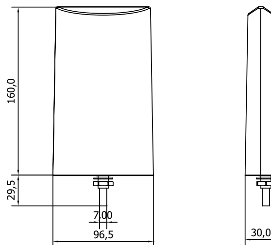
Fig. 4 Dimensions antenne
