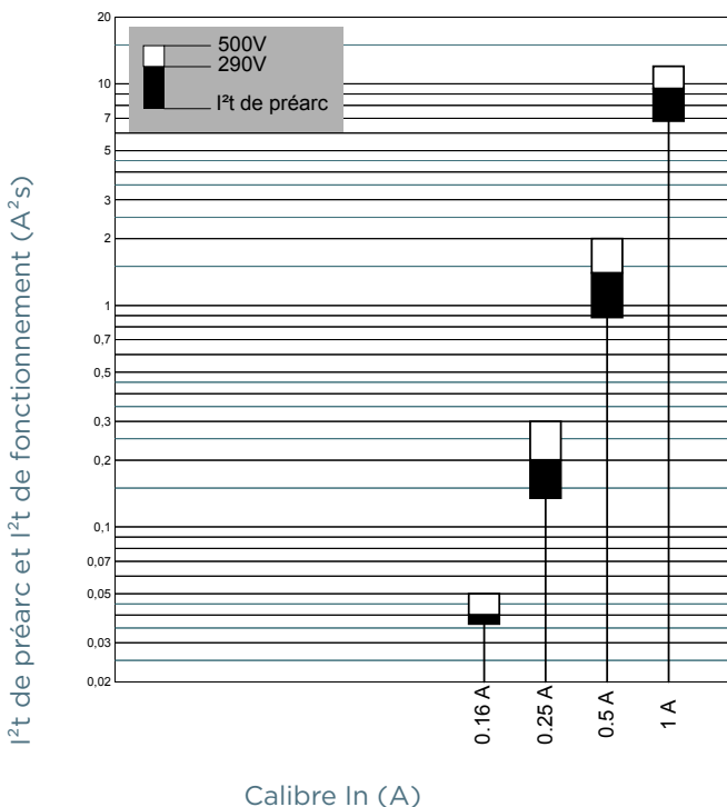
Taille 10x38 500V aM sans percuteur
