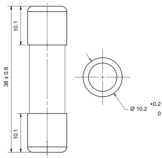
Taille 10x38 aM sans indicateur (1001210)
