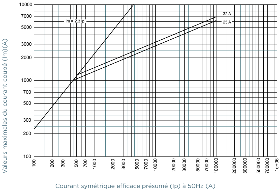
Taille 10x38 250V aM avec percuteur
